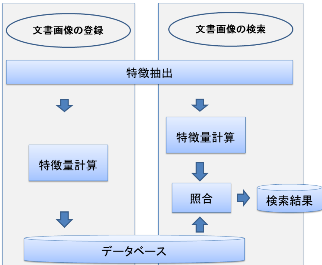
図 3.1: LLAH の処理の概要
