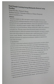
図 1: 文書画像
