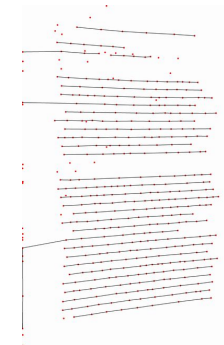
図 2: 単語の並び
